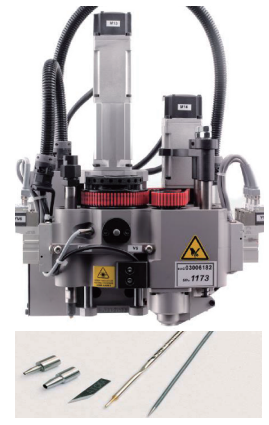
配屬5或7工具 5- OR 7-TOOL CUTTING HEAD
